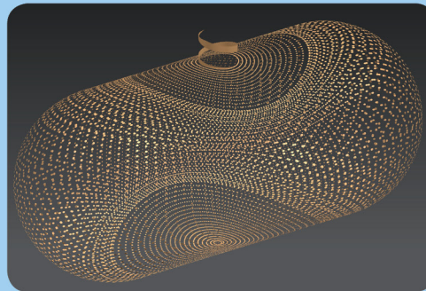
【智能三维清洗喷头】清洗轨迹图
