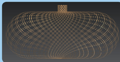
【传统三维清洗喷头】清洗轨迹图
