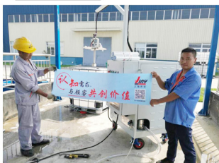
吨桶高压清洗系统
