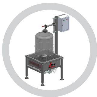
开口桶清洗
