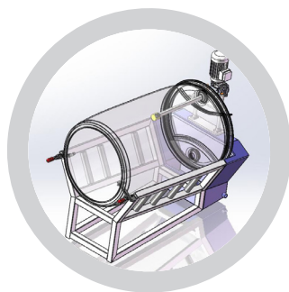
小口桶清洗
