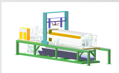
压滤机清洗系统
